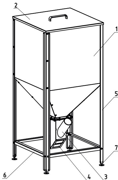
Рис.4 Топливный бункер
